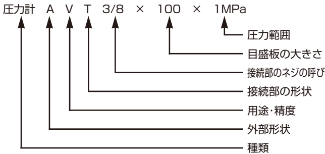
圧力計
